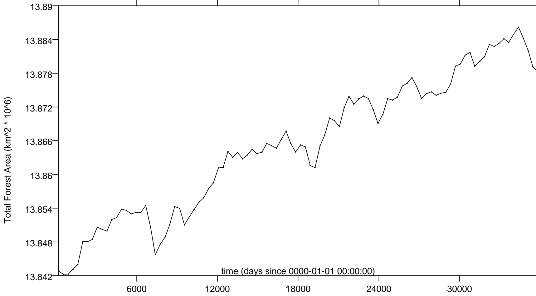
Forest_area_pmip2_0k_oav
