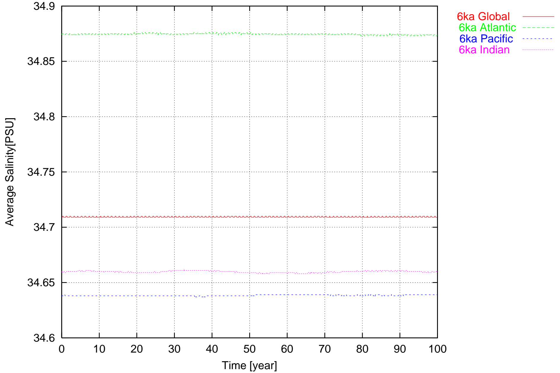
6ka Ocean SSS Trend
