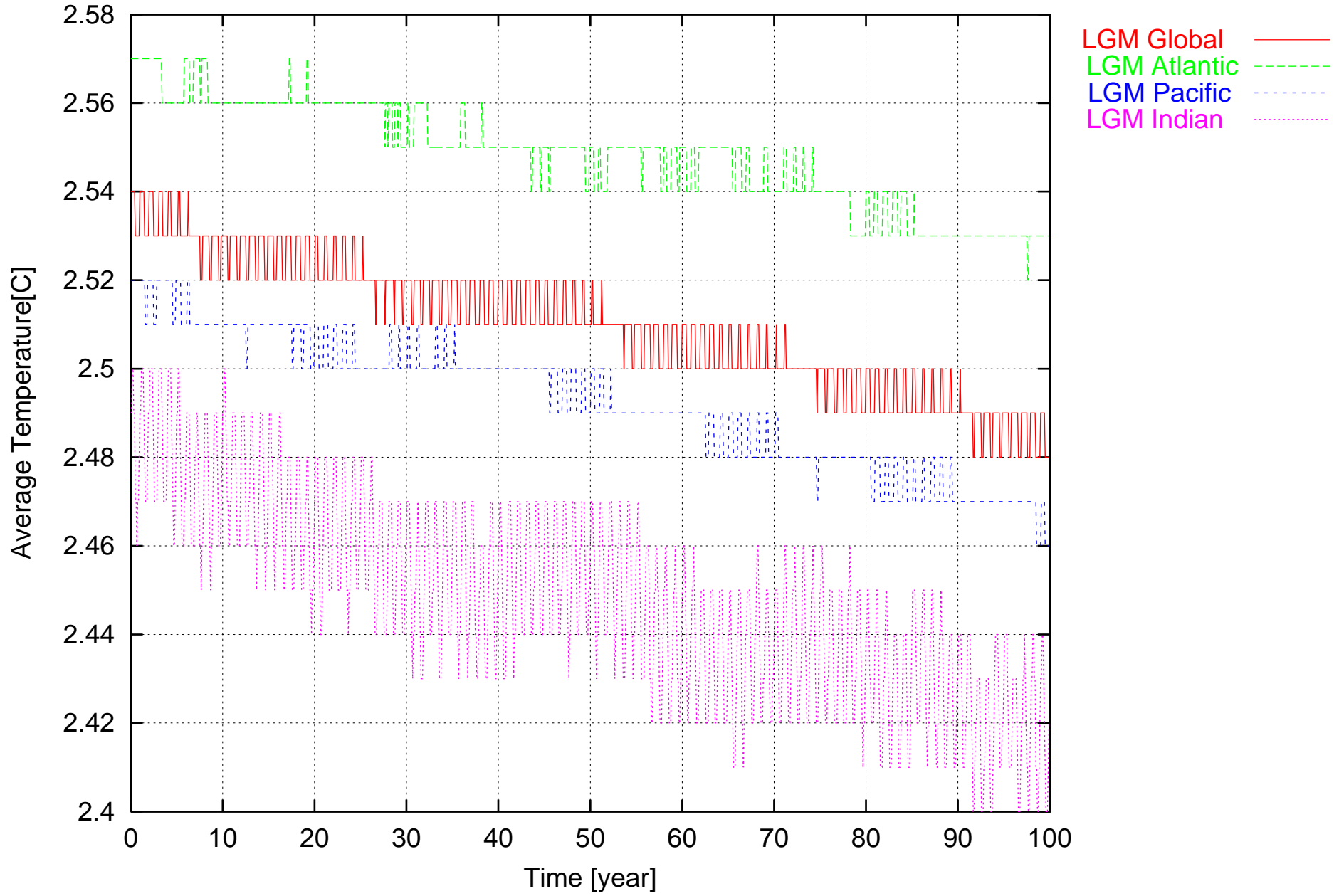
LGM Ocean SST Trend
