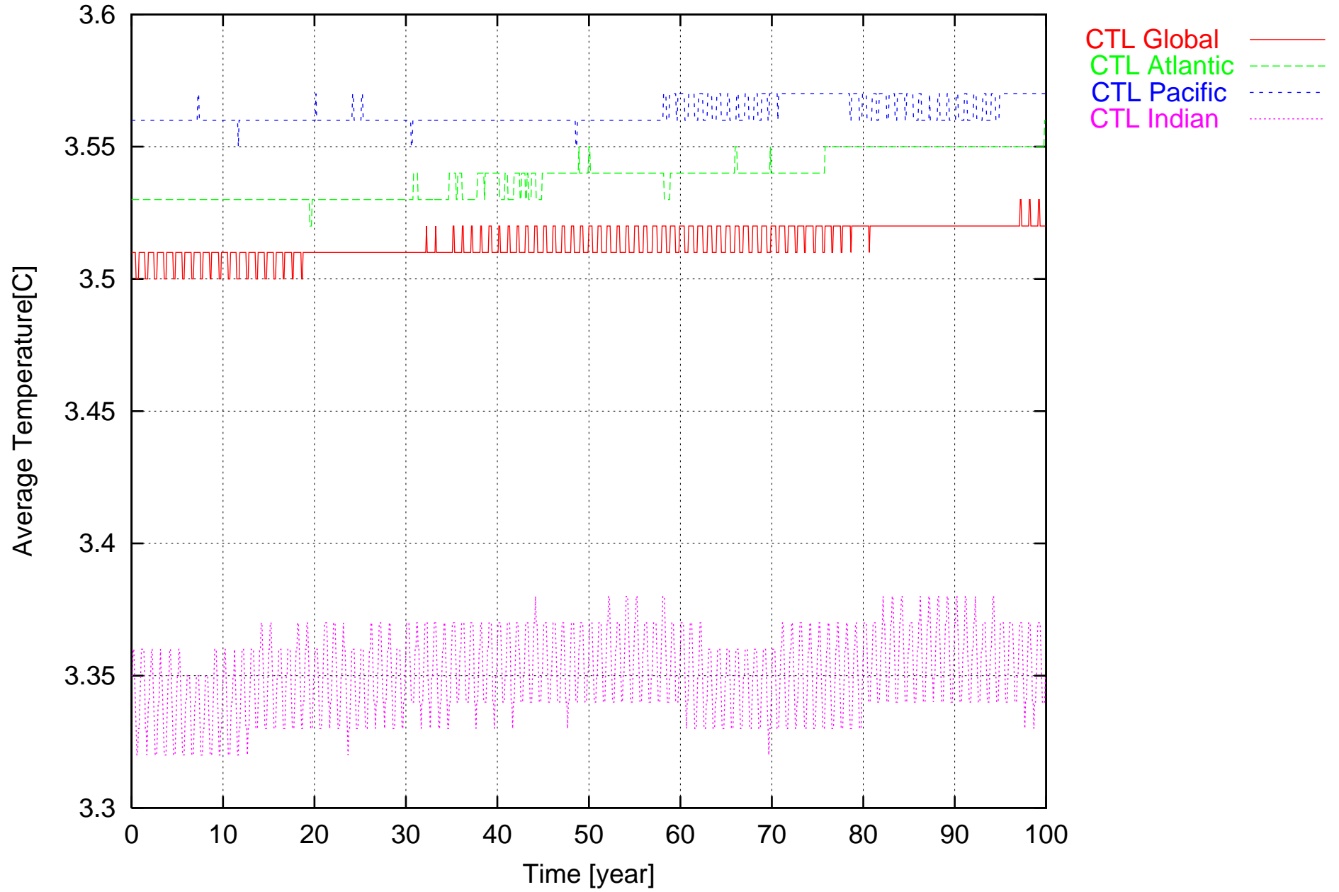
CTL Ocean SST Trend
