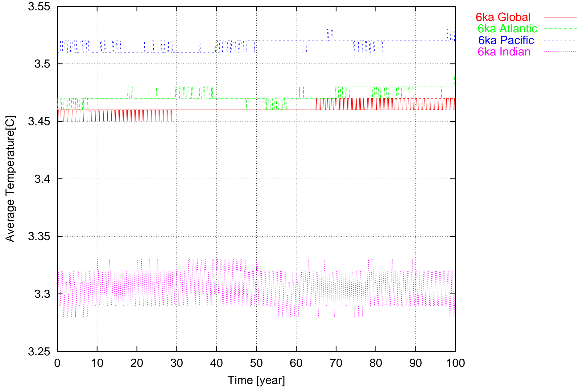
6ka Ocean SST Trend
